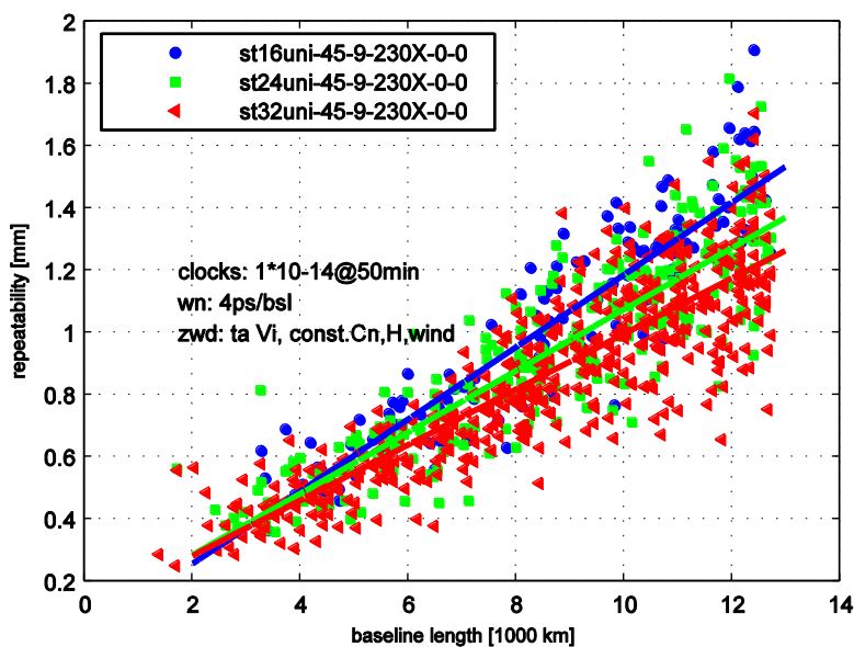
Abb. 6-24: Basislinienlängen-Wiederholbarkeit ( repeatability ) für die drei V2C-Testnetzwerke mit 16 (blau), 24 (grün) und 32 (rot) VLBI-Stationen. Zur Erstellung des Beobachtungsplanes wurde der uniform sky Algorithmus mit einer Beobachtungsdauer von 45 s verwendet. Der MCS verwendete ein stationsunabhängiges Turbulenzmodell mit konstanten Werten für C_n , H und der Windgeschwindigkeit.
