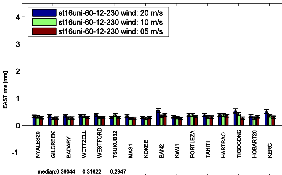
Abb. 5-31: RMS der Ostkomponente ( East ) der 3D-Stationsposition in der Stationsreihenfolge von Nord nach Süd. Die Atmosphäre wurde mit dem Vienna Turbulenzmodell und Windgeschwindigkeiten von 20 m/s (blau), 10 m/s (grün) und 5 m/s (braun) in Richtung Osten simuliert.
