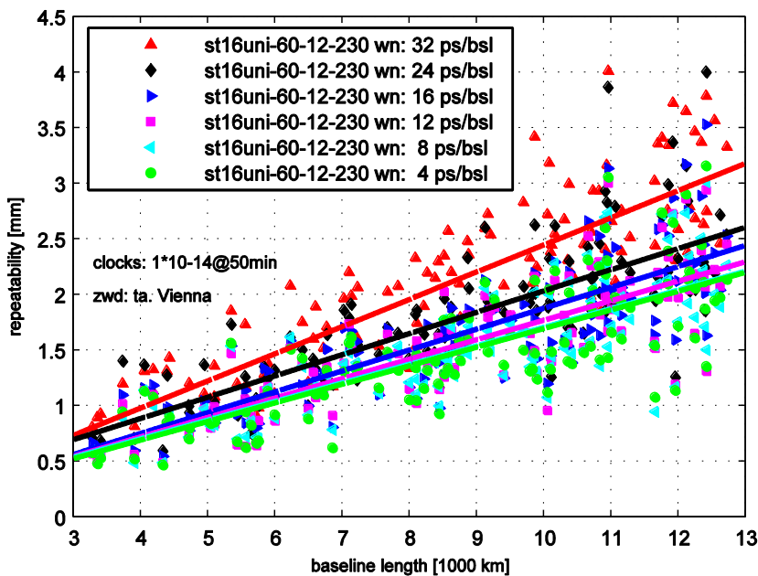
Abb. 5-42: Basislinienlängen-Wiederholbarkeit ( repeatability ) für den 16 Stationen uniform sky Beobachtungsplan mit einem Beobachtungsintervall von 60 s. Das weiße Rauschen wurde mit 32 ps (rot), 24 ps (schwarz), 16 ps (blau), 12 ps (magenta), 8 ps (türkis) und 4 ps (grün) simuliert.
