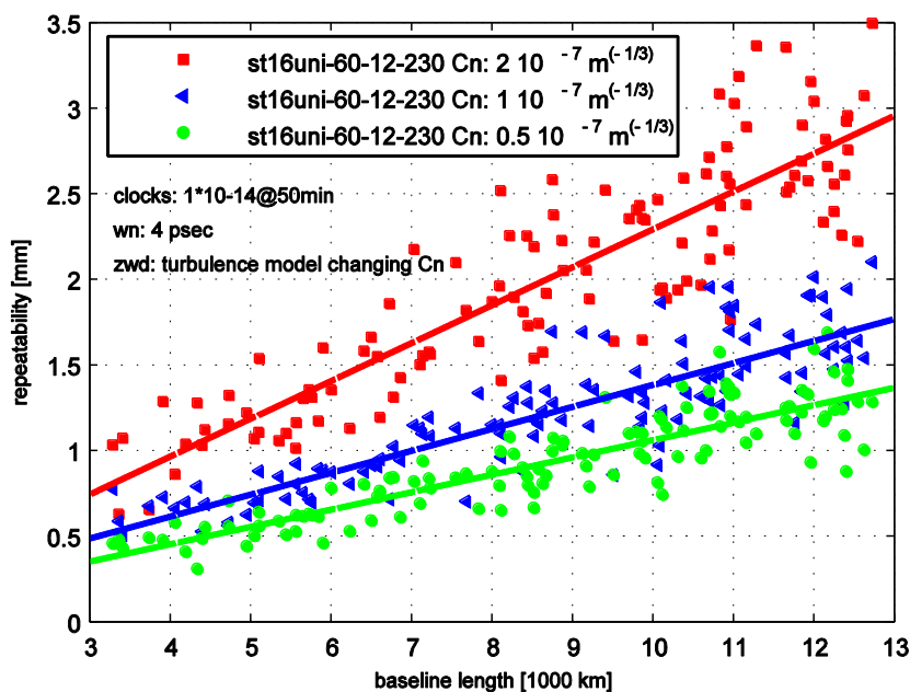
Abb. 5-16: Basislinienlängen-Wiederholbarkeit ( repeatability ) für den 16 Stationen uniform sky Beobachtungsplan mit einem Beobachtungsintervall von 60 s. Für die Simulation der Atmosphäre mit dem Vienna Turbulenzmodell wurden Cn-Werte von 0.5 \cdot 10^{-7} \text{ m}^{-1/3} (grün), 1 \cdot 10^{-7} \text{ m}^{-1/3} (blau) und 2 \cdot 10^{-7} \text{ m}^{-1/3} (rot) verwendet.
