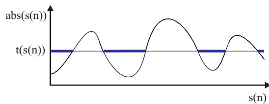
(b) LoLAS
