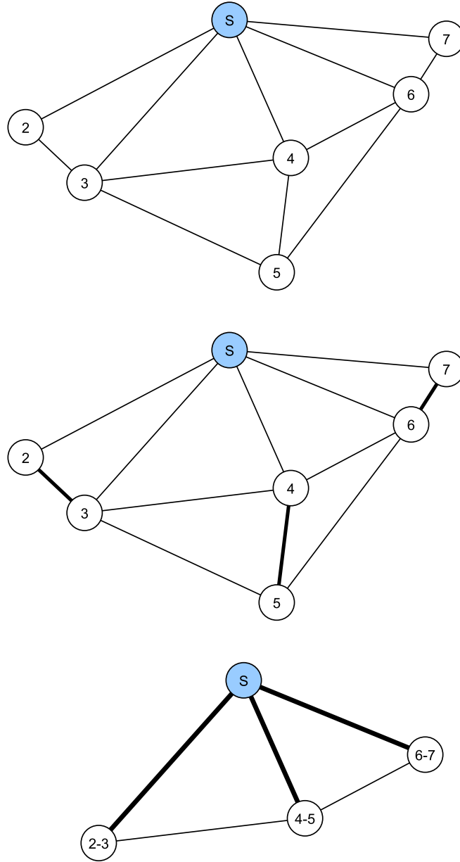
Abbildung 4.2: Das Coarsening. Der Graph wird sukzessive vereinfacht, indem Knoten zusammengefasst werden.
