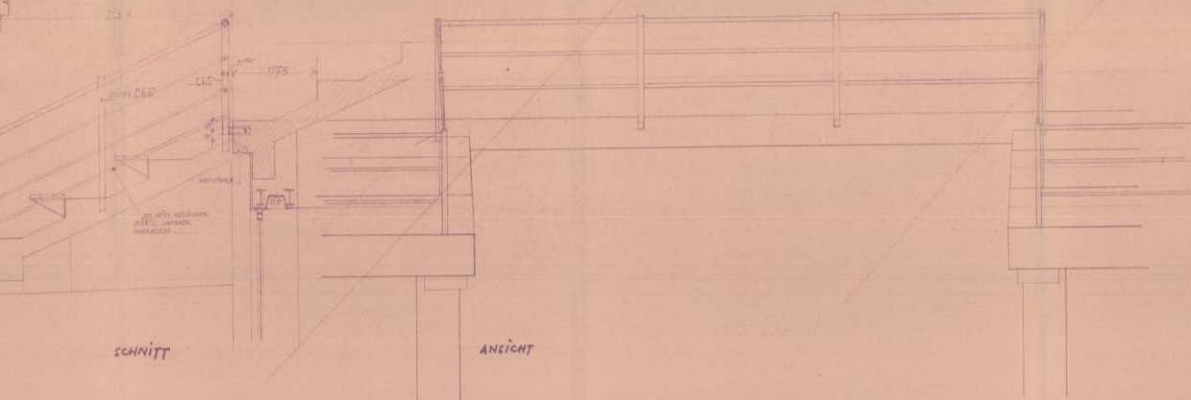
GELÄNDER ZWISCHEN RAHMEN 172-1 BEI ZUGANG ZUR EHRENLOGE, M=1:20
