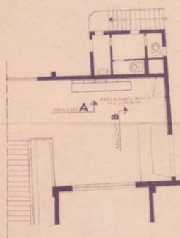
GRUNDRISS M=1:100
