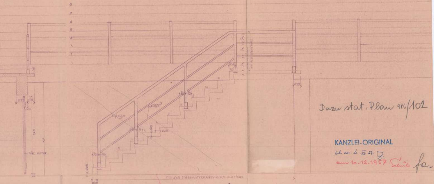
ANSICHT B M = 1:20
