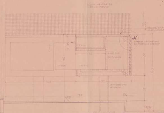
SNITT A-A
