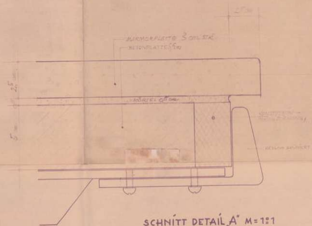
SCHNITT DETAIL A M 1:1
