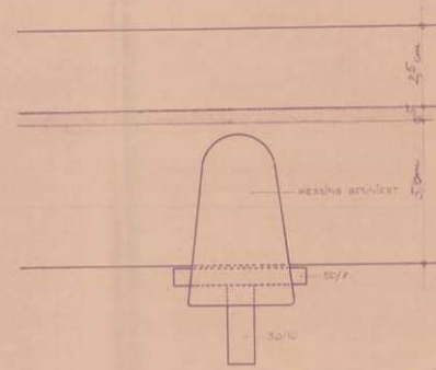
ANSICHT DETAIL A M 1:1
