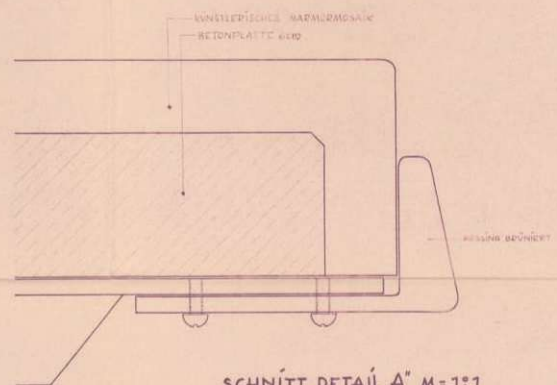
SCHNITT DETAIL "A" M 1:1
