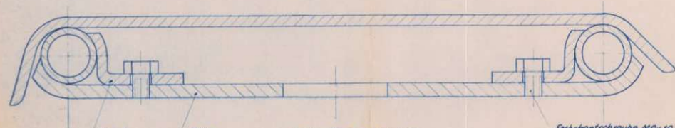
Schnitt C-D (M.: 1:1)
