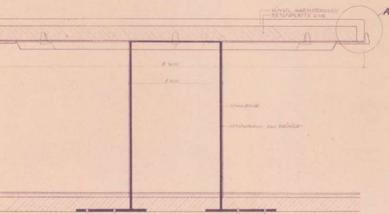
SCHNITT M 1:5
