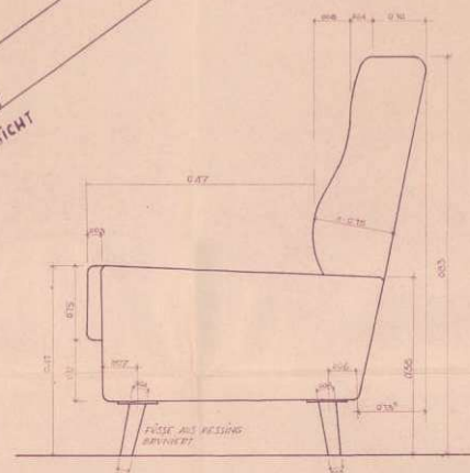
SEITENANSICHT SITZBANK
