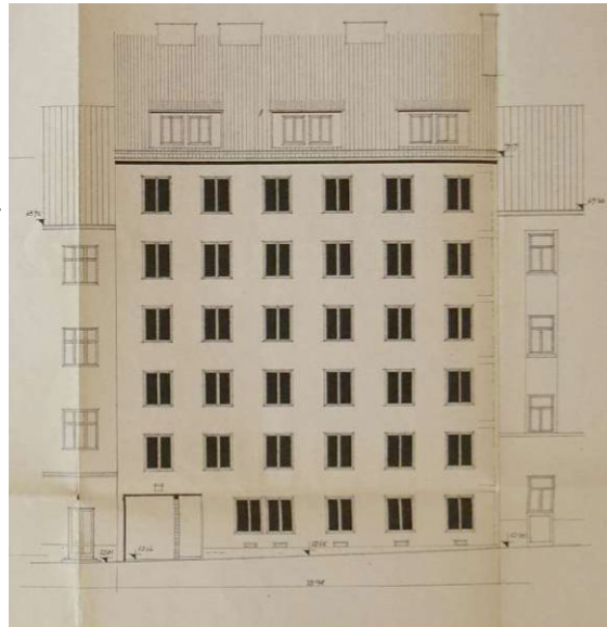
18 MA 37, Ansicht Waldgasse, Auswechselungsplan 1959
