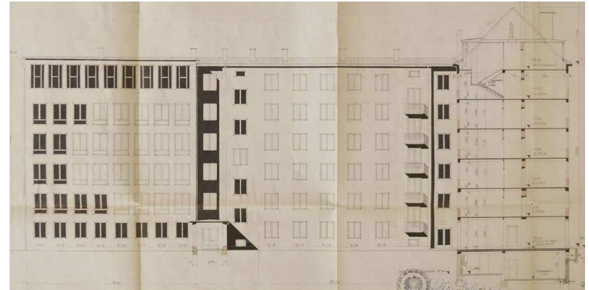
20MA 37, Ansicht und Schnitt Hof, Auswechselungsplan 1959
