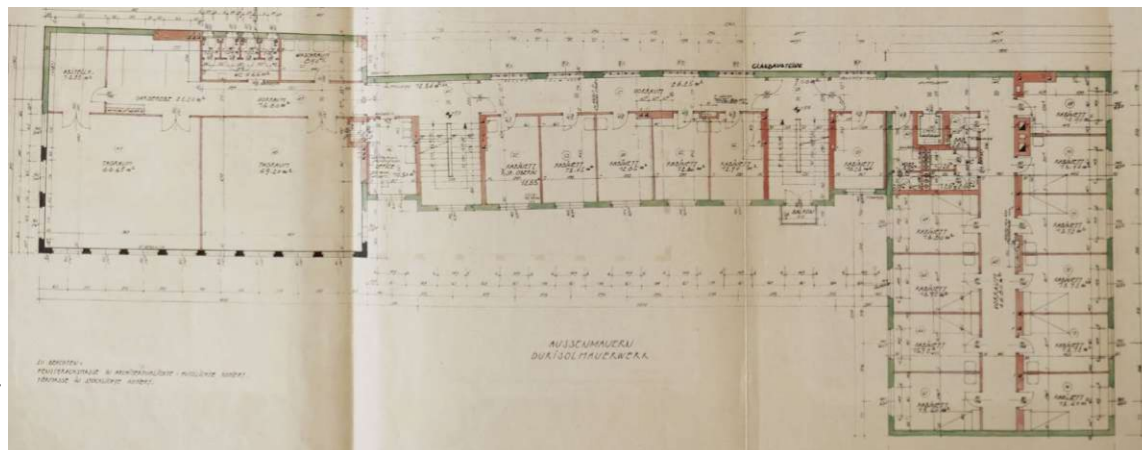
14 MA 37, Grundriss 1.Obergeschoss, Auswechselungsplan 1959
