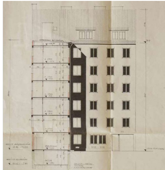
19 MA 37, Ansicht und Schnitt Gellertplatz, Auswechselungsplan 1959
