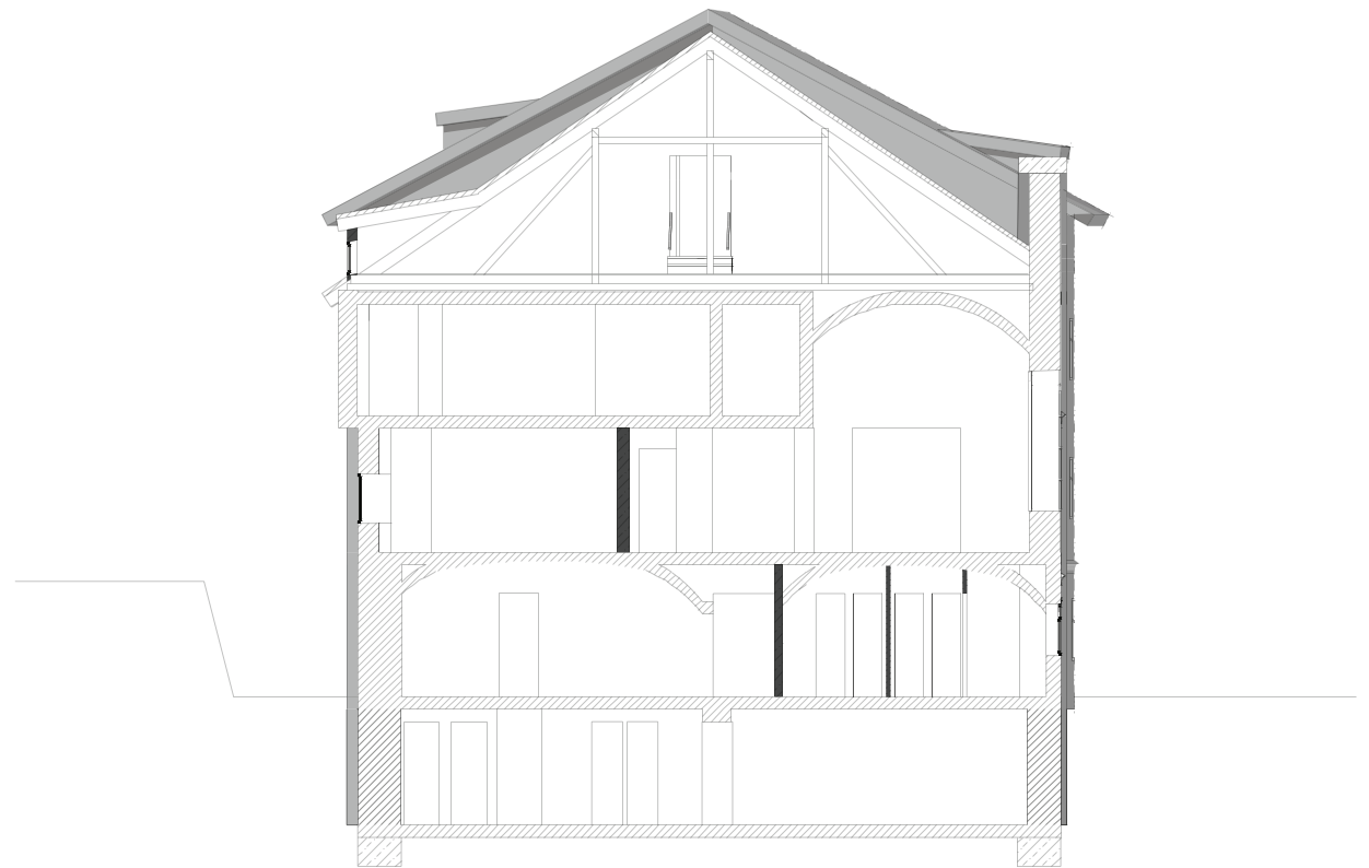
Abb.42 Schnitt B-B
