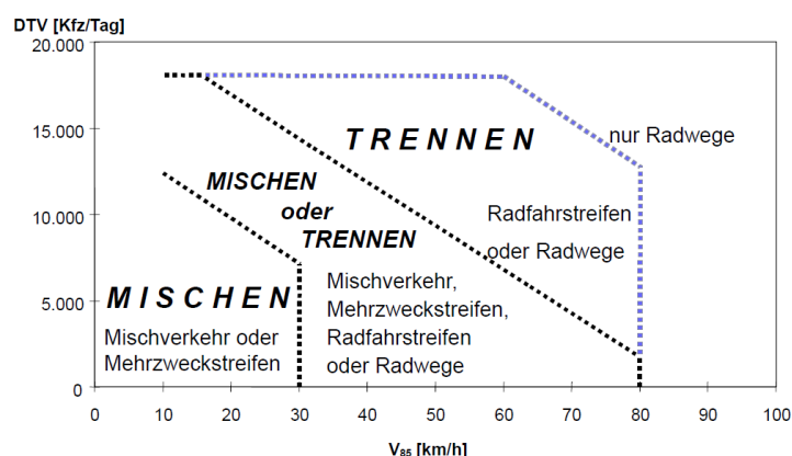
Abb. 15: Mischung- bzw. Trennung von Rad- und Kfz-Verkehr (Quelle: FSV, 2014b: 13)
