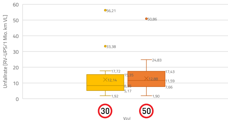
Abb. 72: Unfallraten der ausgewählten Streckenabschnitte nach höchstzulässiger Fahrgeschwindigkeit, 2013-2016; eigene Darstellung (Datenquelle: KfV Verkehrsunfallstatistik - Statistik Austria; Nast Consulting; Stadt Wien - data.wien.gv.at, 2017: online; Stadt Wien - ViennaGIS, 2017: online; Stadt Wien MA 18, 2016: online; eigene Erhebung)
