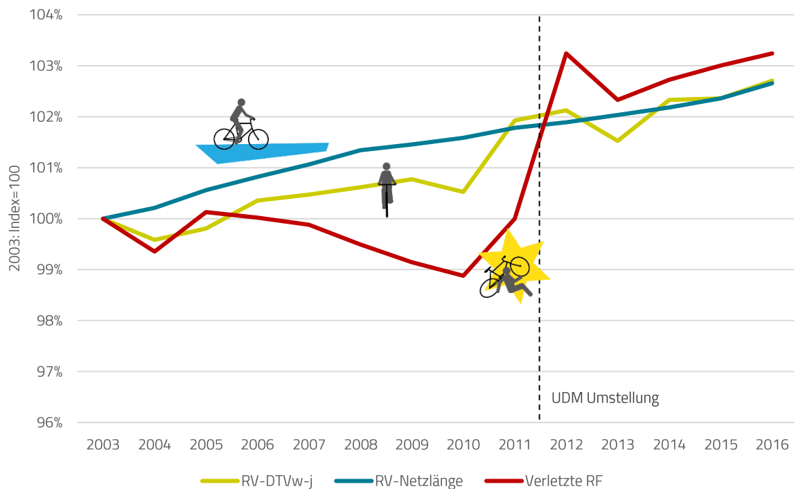
Abb. 69: Zusammenhang zwischen Verkehrsleistung (RV-DTVw-j), Länge des Radverkehrsnetzes und verletzten Radfahrenden in Wien, 2003–2016; eigene Darstellung (Datenquelle: KfV Verkehrsunfallstatistik - Statistik Austria; Nast Consulting; Mobilitätsagentur Wien)
