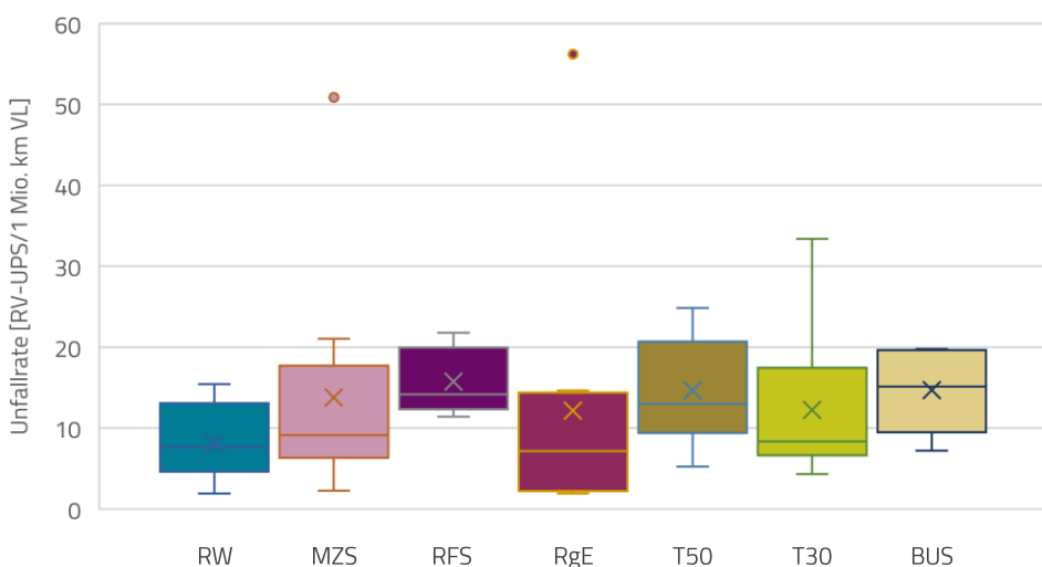
Abb. 78: Unfallraten der ausgewählten Streckenabschnitte nach RVA, 2013-2016; eigene Darstellung (Datenquelle: KFV Verkehrsunfallstatistik - Statistik Austria; Nast Consulting; Stadt Wien - data.wien.gv.at, 2017: online; Stadt Wien - ViennaGIS, 2017: online; Stadt Wien MA 18, 2016: online; eigene Erhebung)
