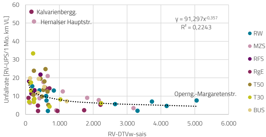
Abb. 75: Scatterplot der Unfallraten der ausgewählten Streckenabschnitte und des RV-DTVw-sais, 2013-2016; eigene Darstellung (Datenquelle: KfV Verkehrsunfallstatistik - Statistik Austria; Nast Consulting; Stadt Wien - data.wien.gv.at, 2017: online; Stadt Wien - ViennaGIS, 2017: online; Stadt Wien MA 18, 2016: online; eigene Erhebung)
