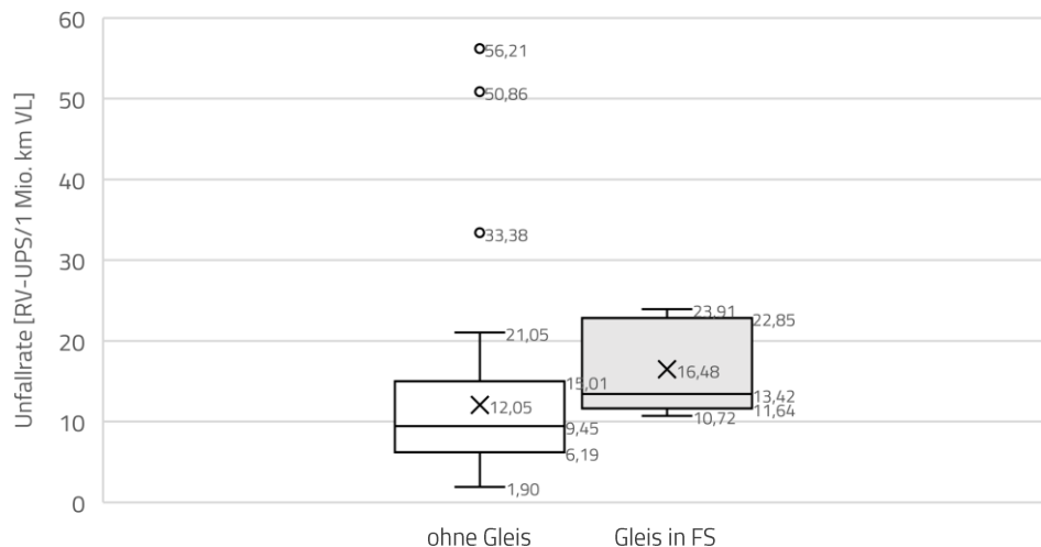
Abb. 73: Unfallraten der ausgewählten Streckenabschnitte nach der FS-Führung auf Gleis, 2013-2016; eigene Darstellung (Datenquelle: KfV Verkehrsunfallstatistik - Statistik Austria; Nast Consulting; Stadt Wien - data.wien.gv.at, 2017: online; Stadt Wien - ViennaGIS, 2017: online; Stadt Wien MA 18, 2016: online; eigene Erhebung)
