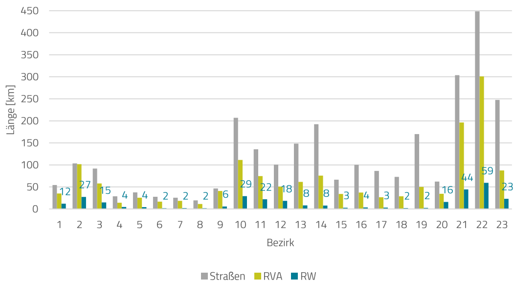
Abb. 28: Länge der öffentlichen Straßen, Radverkehrsanlagen (RVA) und Radwegen (RW) in den Wiener Gemeindebezirken 2016; eigene Darstellung (Datenquelle: Stadt Wien MA 28 & MA 46, 2017: online)
