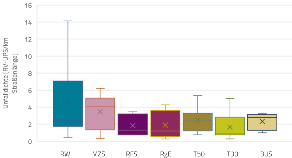
Abb. 77: Unfalldichten der ausgewählten Streckenabschnitte nach RVA, 2013-2016; eigene Darstellung (Datenquelle: KFV Verkehrsunfallstatistik - Statistik Austria; Nast Consulting; Stadt Wien - data.wien.gv.at, 2017: online; Stadt Wien - ViennaGIS, 2017: online; Stadt Wien MA 18, 2016: online; eigene Erhebung)
