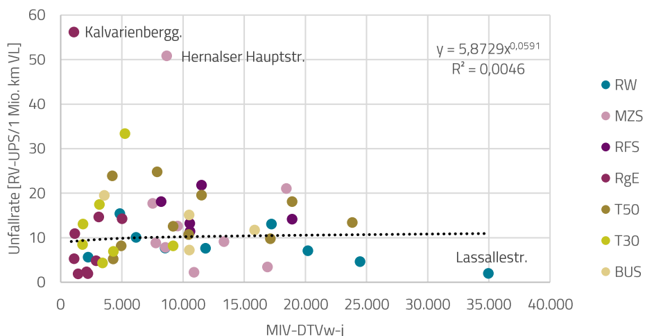
Abb. 74: Scatterplot der Unfallraten der ausgewählten Streckenabschnitte und des MIV-DTVw-j, 2013-2016; eigene Darstellung (Datenquelle: KfV Verkehrsunfallstatistik - Statistik Austria; Nast Consulting; Stadt Wien - data.wien.gv.at, 2017: online; Stadt Wien - ViennaGIS, 2017: online; Stadt Wien MA 18, 2016: online; eigene Erhebung)
