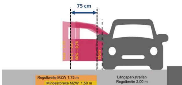
Abb. 79: Vergleich Türöffnungsbreite (Dooring Zone) und Regel- und Mindestbreite von MZS (Quelle: Szeiler & Skoric, 2017: 4)
