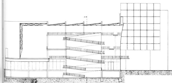
SCHNITT 11
