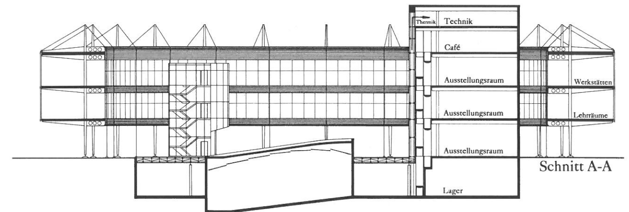
Ost-Ansicht
